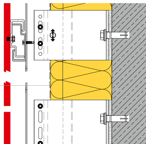
DETALLE CON JUNTA HORIZONTAL A110
