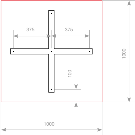
EJEMPLO TABLERO DE MESA SALIENTE Fig. 83
