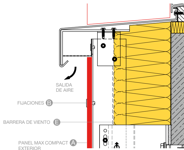
DETALLE INFERIOR DE VENTANA A102
