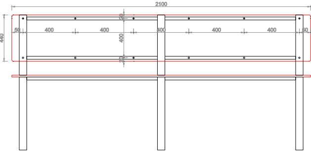
BANCO CON RESPALDO Fig. 86
