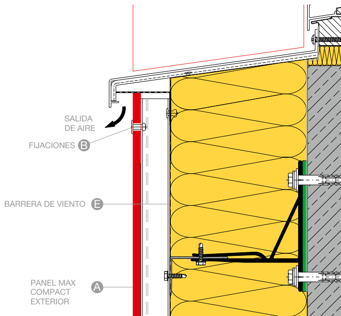
DETALLE INFERIOR DE VENTANA A102
