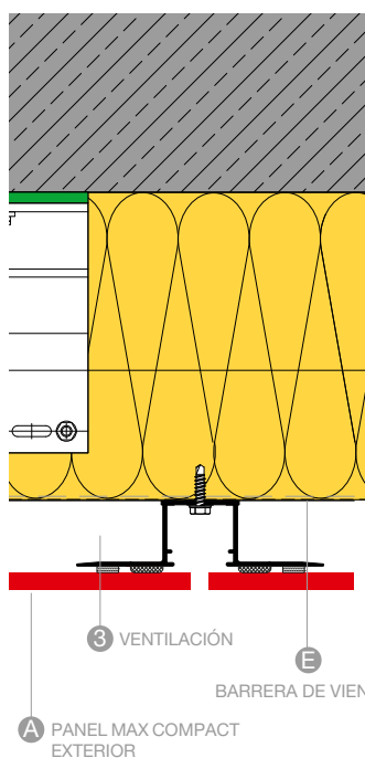
JUNTA VERTICAL A107
