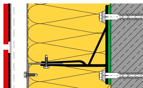
DETALLE CON JUNTA HORIZONTAL A110
