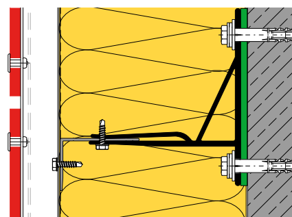
DETALLE CON JUNTA HORIZONTAL A110
