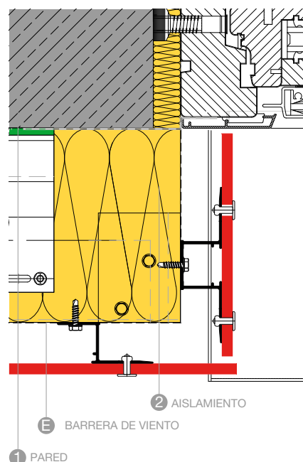
INTRADÓS DE VENTANA A104
