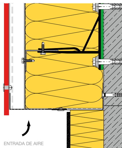
DETALLE CERRAMIENTO INFERIOR A103
