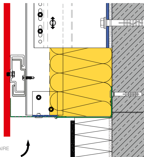
DETALLE CERRAMIENTO INFERIOR A103
