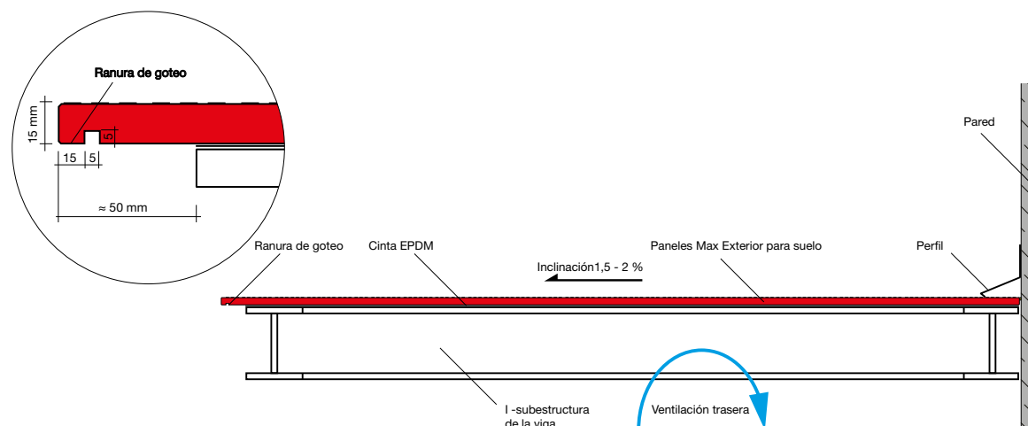
VERTICAL: PRINCIPIO DE VENTILACIÓN E INCLINACIÓN
