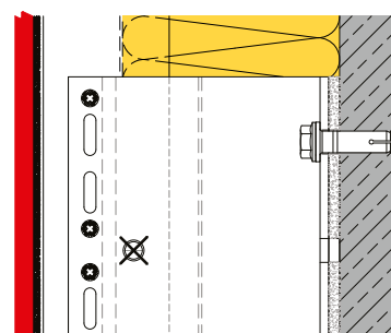
DETALLE CON JUNTA HORIZONTAL A110
