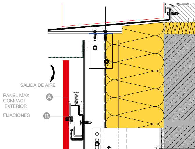
DETALLE INFERIOR DE VENTANA A102
